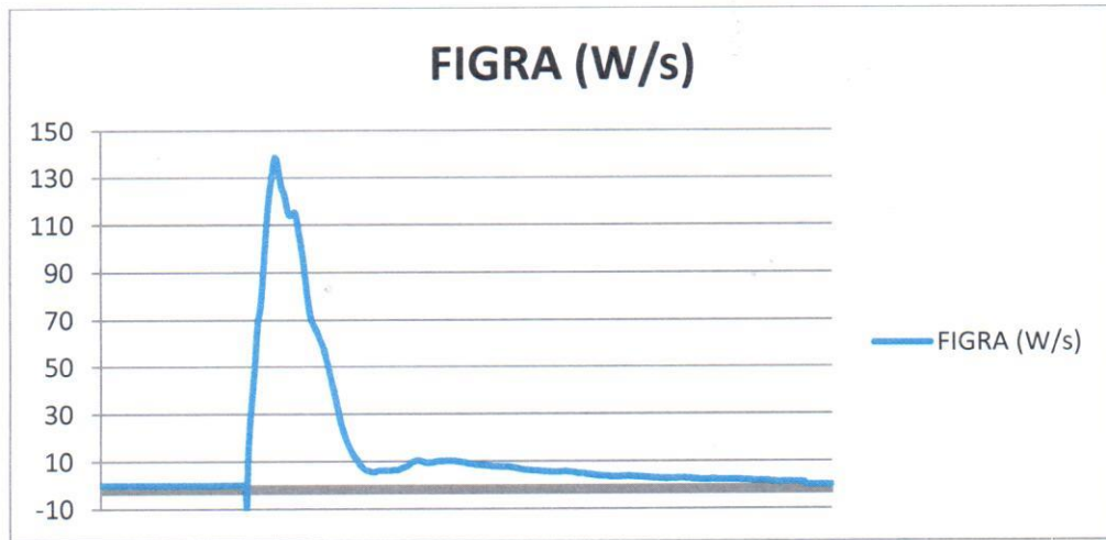
Şekil 2. Numune 1 için 1000 x HRR av (t)/(t-300) değerlerinin grafiği
