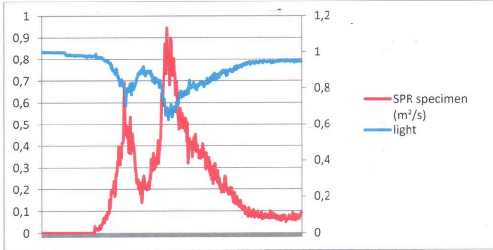
Şekil 6. Numune 2 için SPR_{av}(t) grafiği
