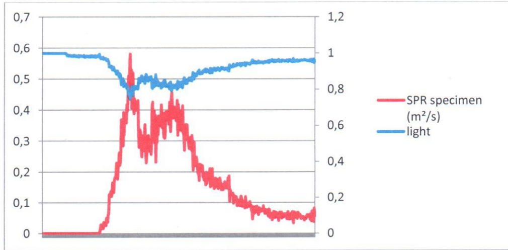
Şekil 3. Numune 1 için SPR_{av}(t) grafiği
